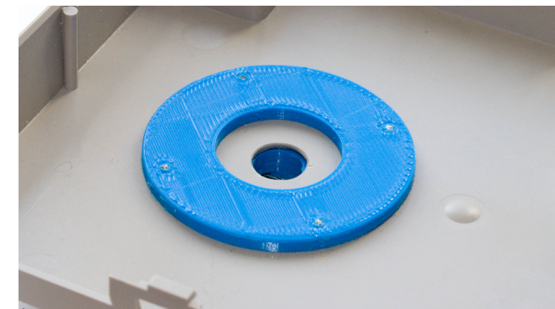
Figuur 13: Contraplaat gemonteerd (voor de opletende lezer: oude versie zonder de verhoging rondom de schroefgaatjes)
