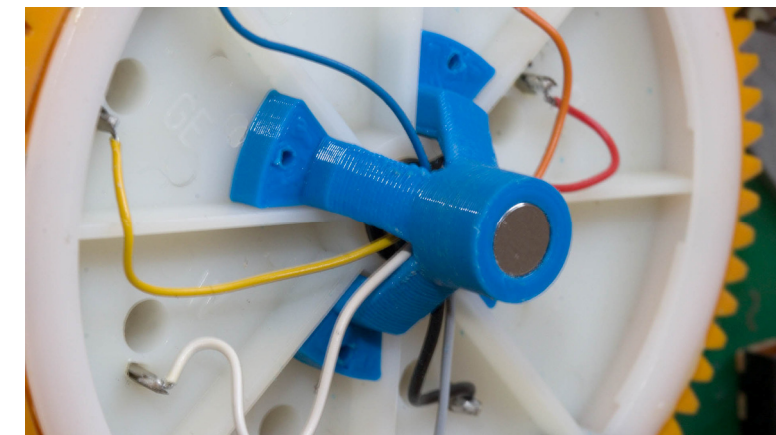
Figuur 5: Magneethouder op schijf plaatsen
