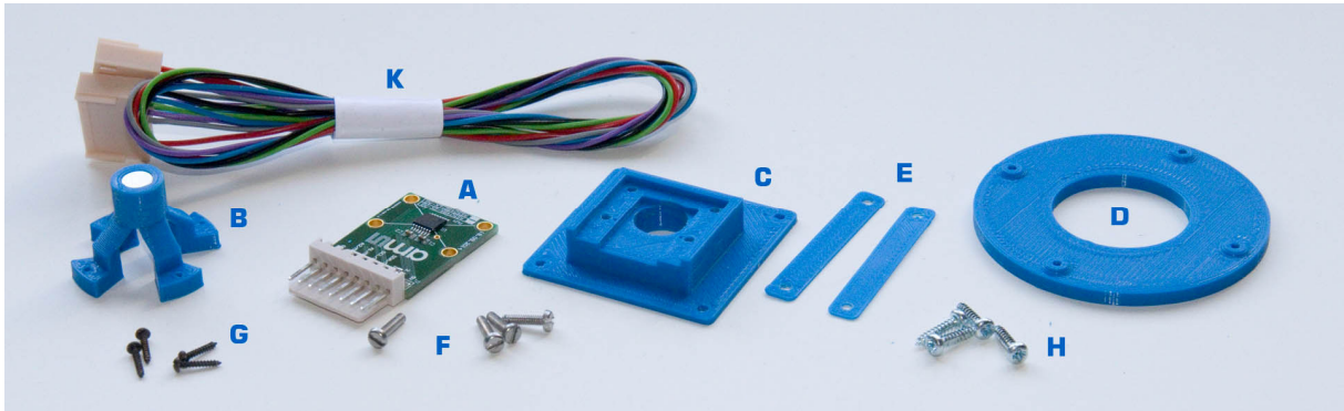
Figuur 1: Onderdelen in het montagepakket
