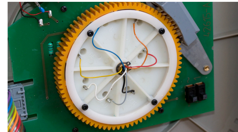
Figuur 4: Schijf met sleepcontacten
