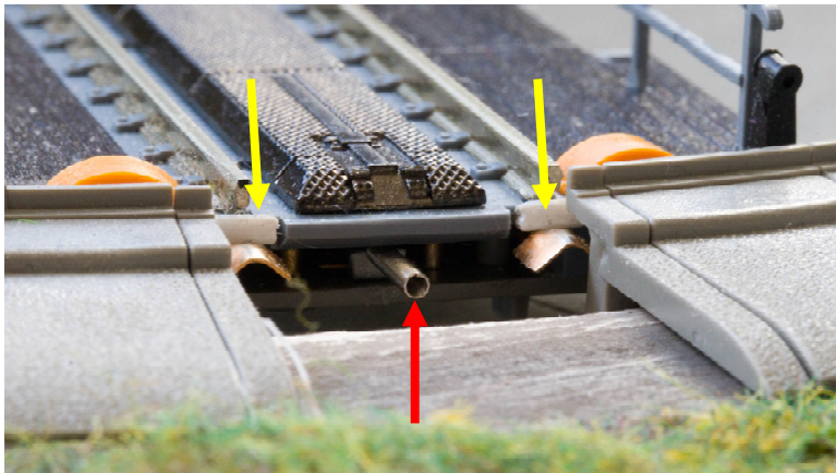
Figuur 17 Geel: Veercontacten geblokkeerd met stukjes polystyreen Rood: Het veertje beschreven in paragraaf 3.3
